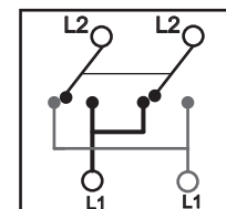
Moduł łączyńca krzyżowego
